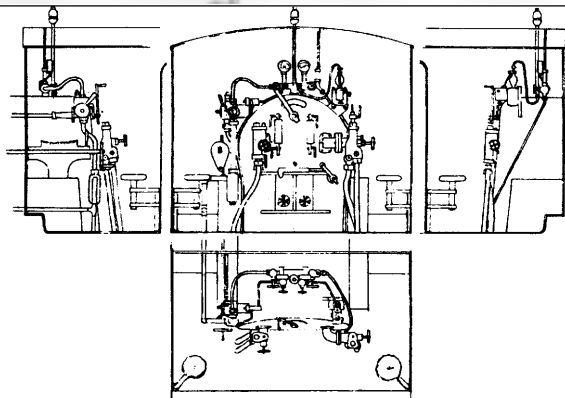
Interiör av en Cc-lokshytt, ritningen i skala HO Foto från Järnvägsmuseum
